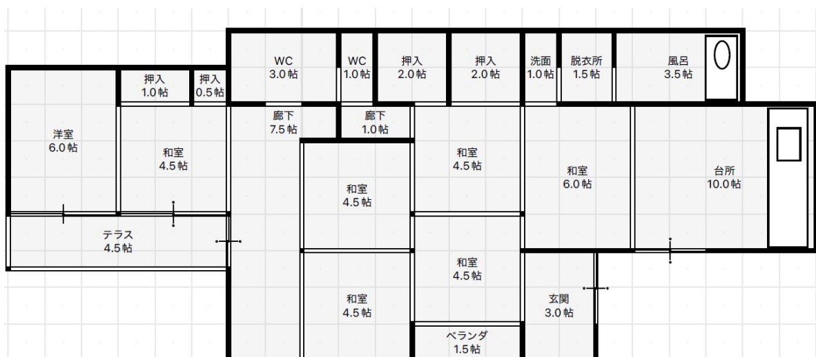
□建物の間取り図
