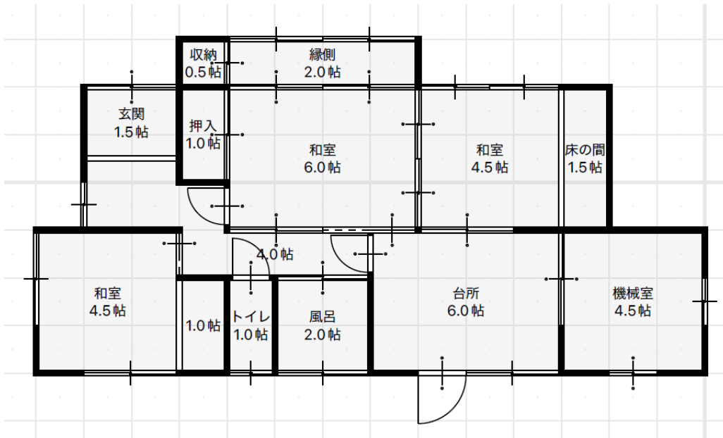
□建物の間取り図
