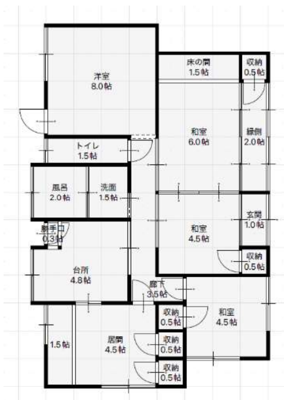
□建物の間取り図
