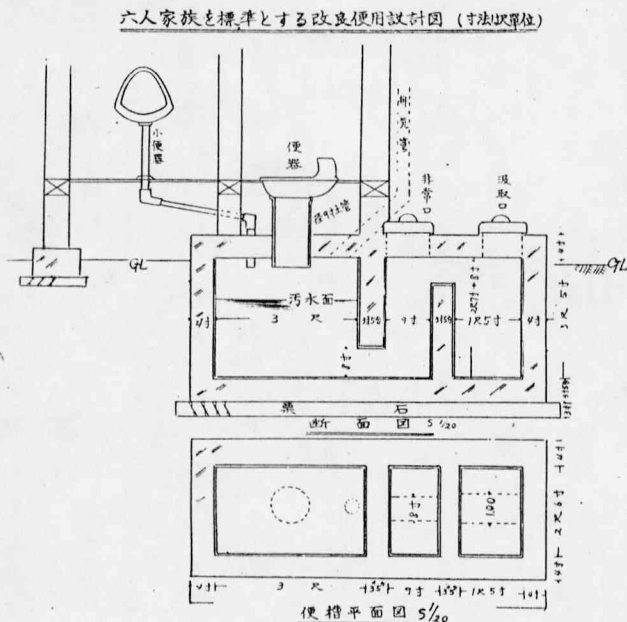
六人家族を標準とする改良便用設計図 (寸法は單位)
