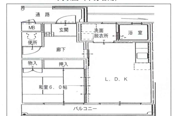
間取図(単身者用)
