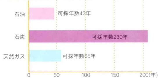
1) 主な化石燃料の可採年数
