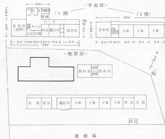
(大原中建築平面図及び配置図)
