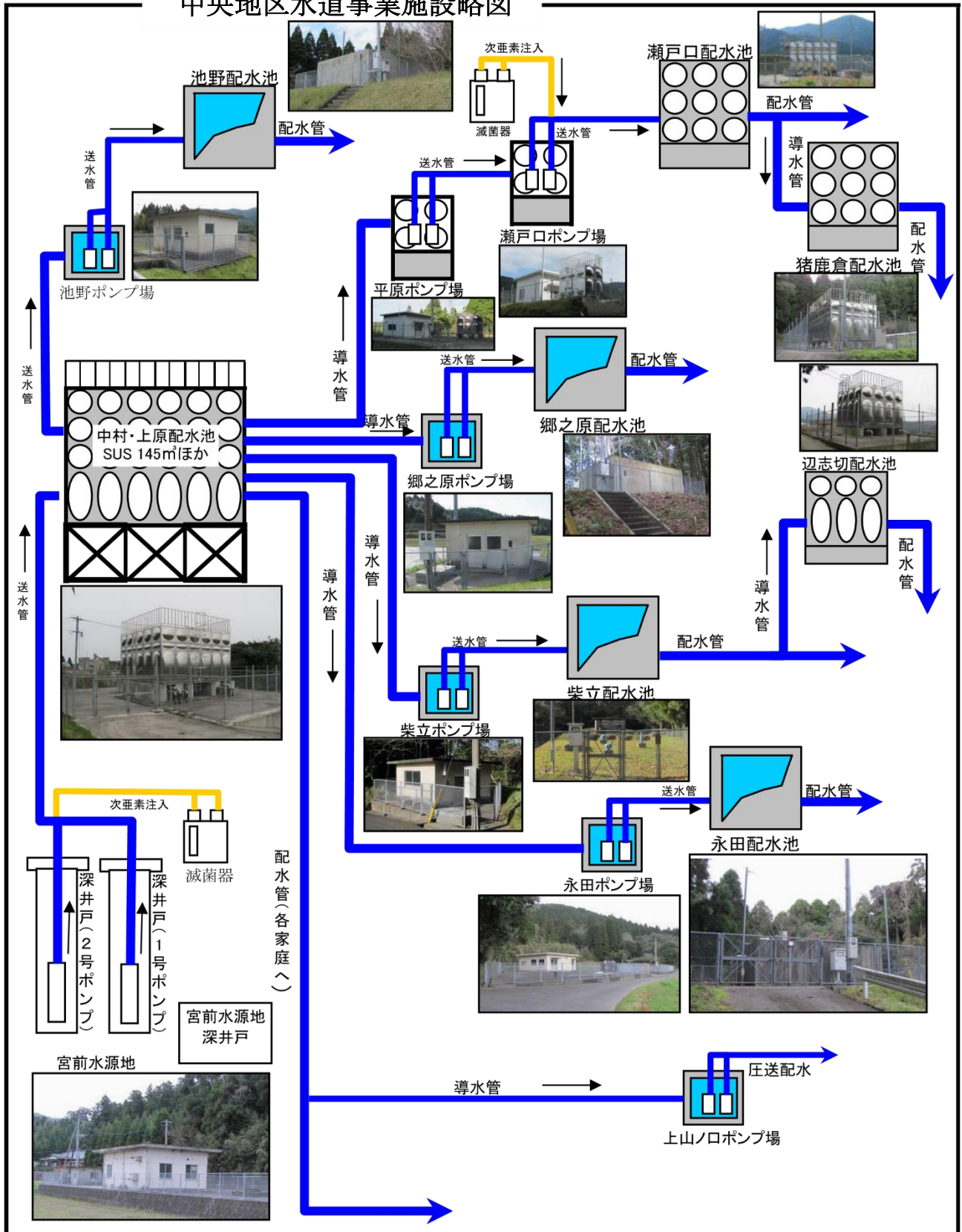
中央地区水道事業施設略図
